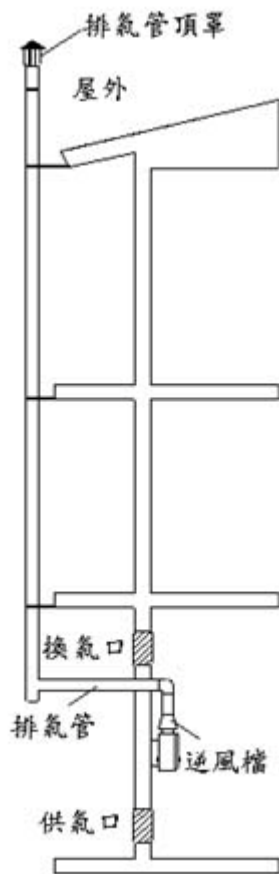
〈圖2〉室內自然排氣型熱水器安裝圖
